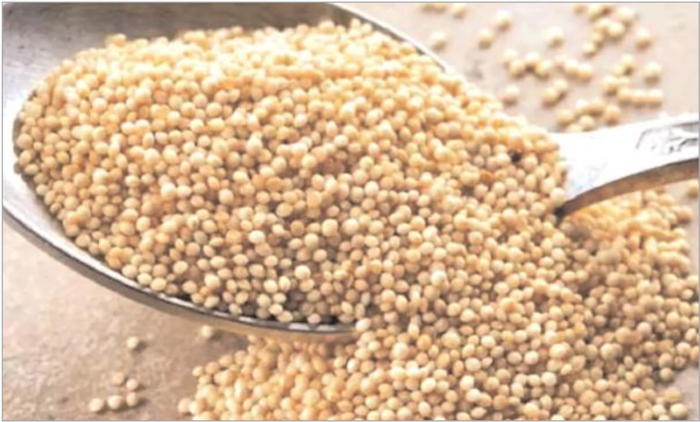
ప్రోటీన్లు
